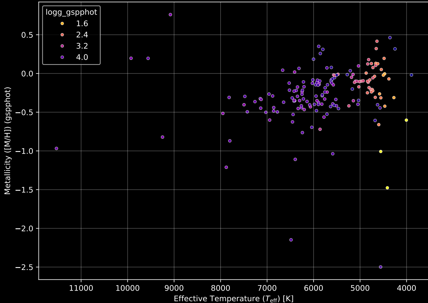
APOGEE DR17 Field: [CVZ_OB02_btx] Stellar Population Parameters (n= 165)
